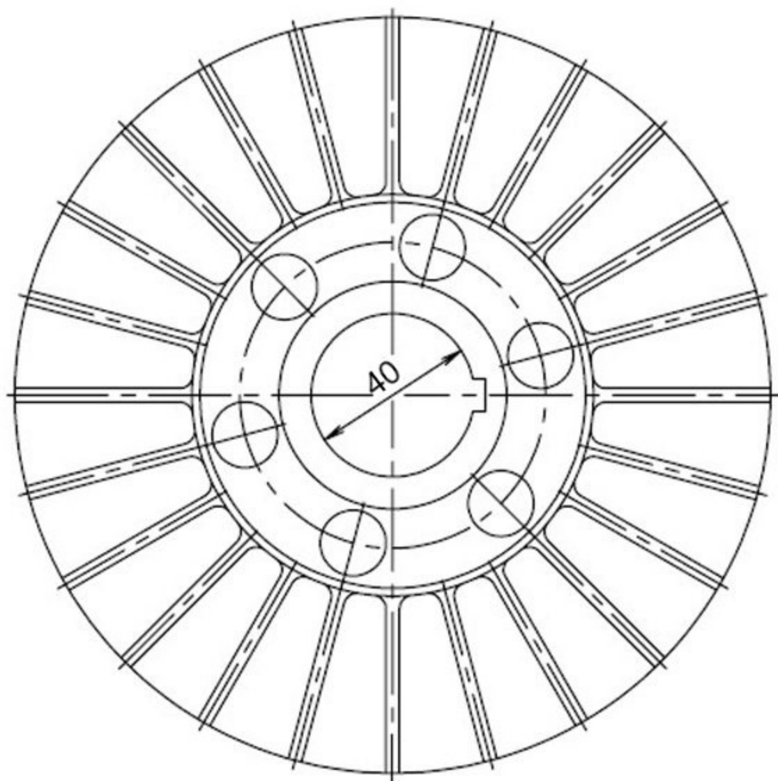
Общий вид колеса вихревого насоса СЦЛ-20-24.
