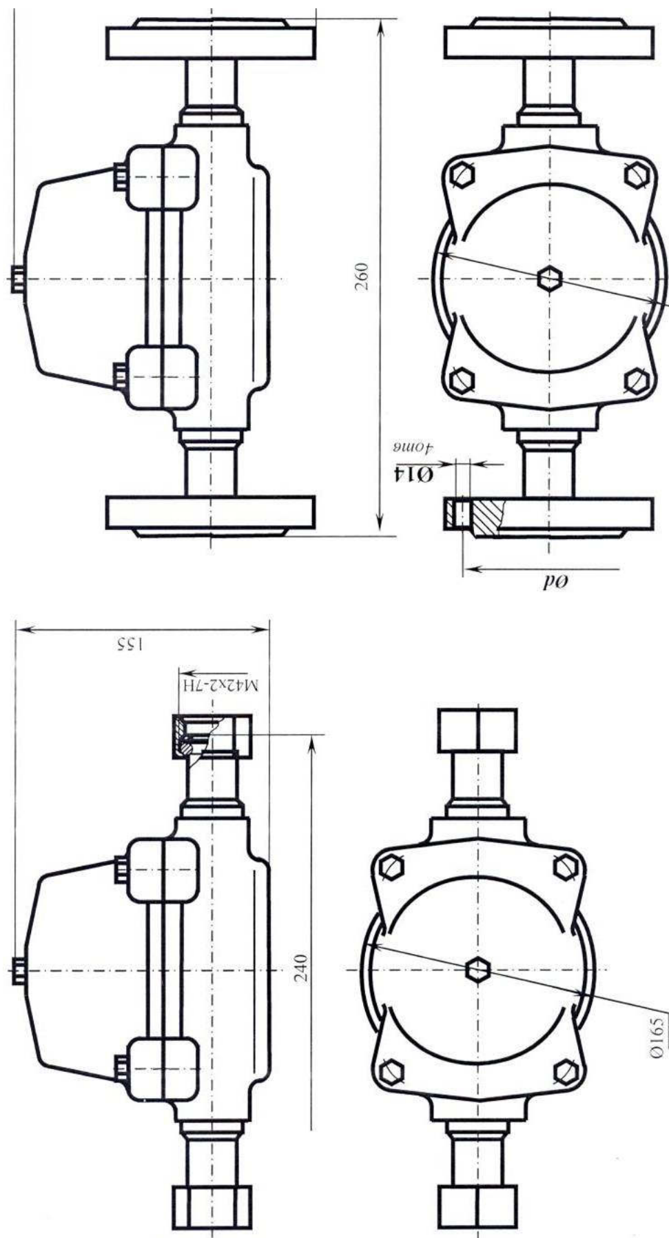
Фильтры жидкости ФЖУ 25-1,6 (литые) Габаритные и присоединительные размеры
