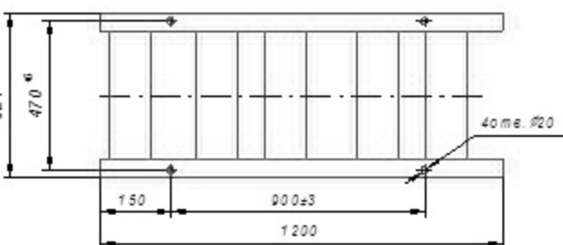
Схема крепления агрегата к фундаменту
