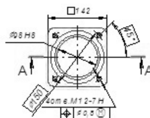
Присоединительные размеры всасывающего фланца
